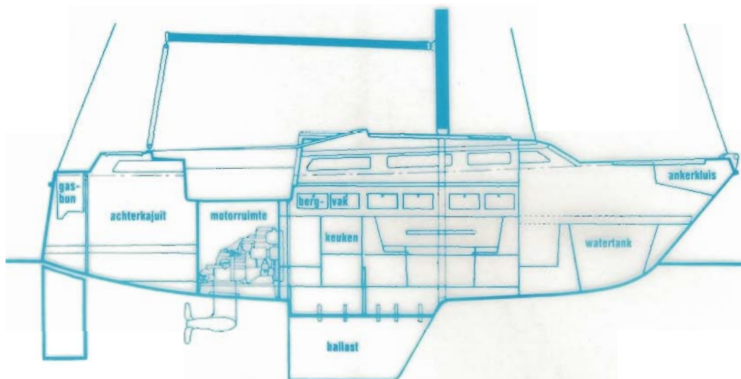
DWARSDOORSNEDE
