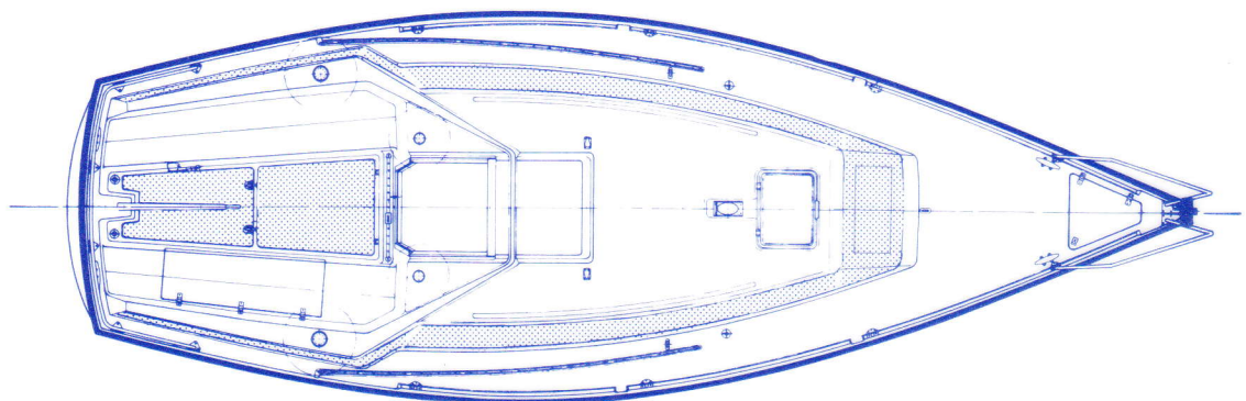
DEKPLAN
