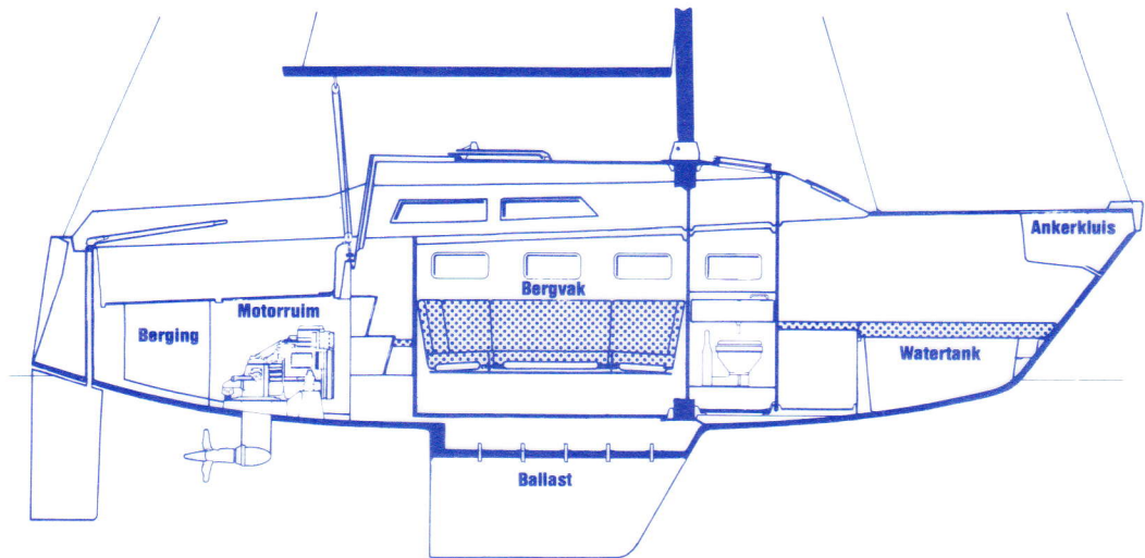
DWARSDOORSNEDE
