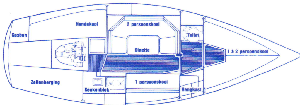
BOVENAANZICHT
