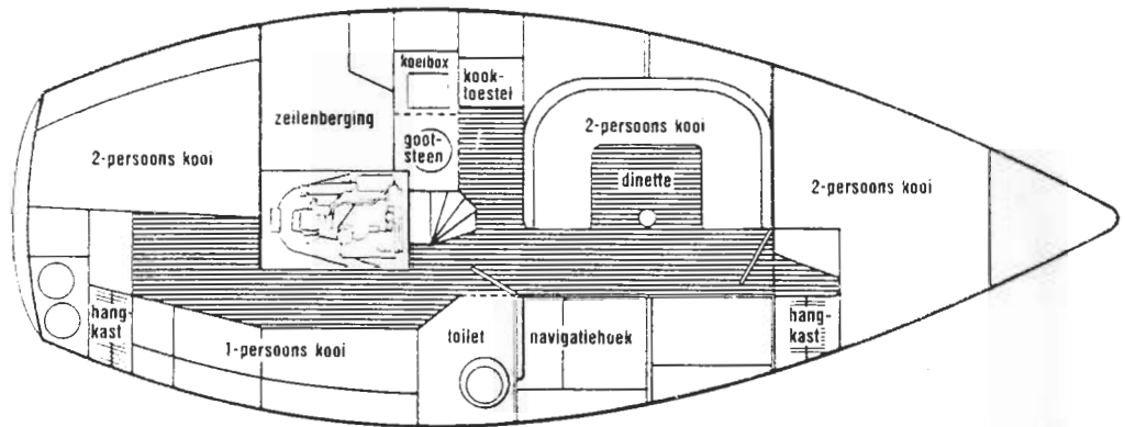
BOVENAANZICHT
