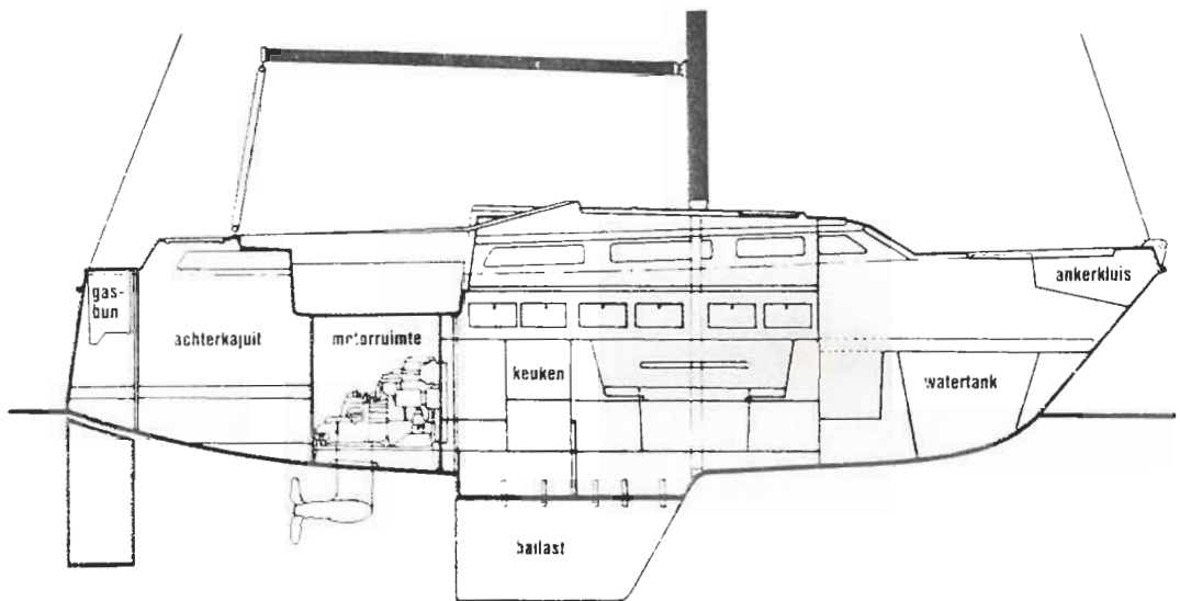
DWARSDOORSNEDE
